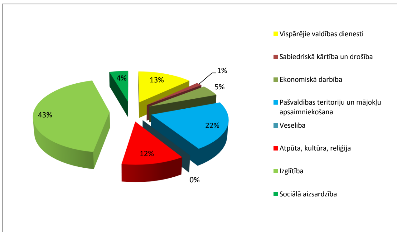
Attēls Nr.2 Beverīnas novada pašvaldības 2017.gada izdevumu sadalījums EUR
