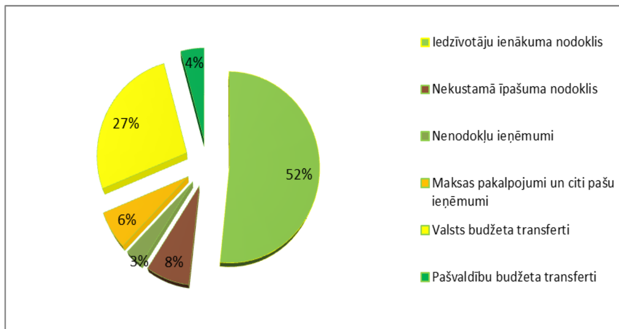
Attēls Nr.1 Beverīnas novada pašvaldības 2017.gada pamatbudžeta ieņēmumu struktūra.
